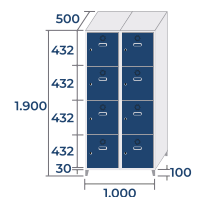
SC-50/2 49,6kg · 0,95m 3
