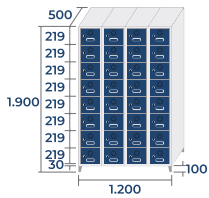
SZ-30/4 85,2kg · 1,14m 3
