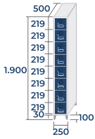
SZ-25/1 23,6kg · 0,24m 3
