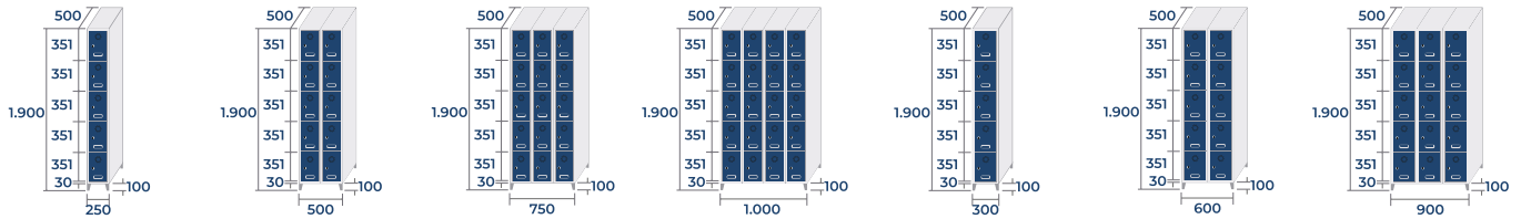
SP-25/1 20,6kg · 0,24m 3 SP-25/2 36,2kg · 0,48m 3 SP-25/3 51,8kg · 0,71m 3 SP-25/4 67,4kg · 0,95m 3 SP-30/1 22kg · 0,29m 3 SP-30/2 39,1kg · 0,57m 3 SP-30/3 56,1kg · 0,86m 3
