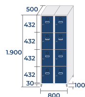
SC-40/2 44kg · 0,76m 3
