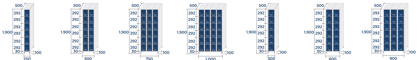
SB-25/1 21,6kg · 0,24m 3 SB-25/2 38,2kg · 0,48m 3 SB-25/3 54,8kg · 0,71m 3 SB-25/4 71,4kg · 0,95m 3 SB-30/1 23kg · 0,29m 3 SB-30/2 41,1kg · 0,57m 3 SB-30/3 59,1kg · 0,86m 3
