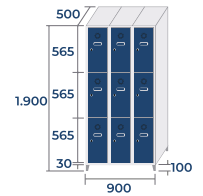
SM-30/3 51kg · 0,86m 3
