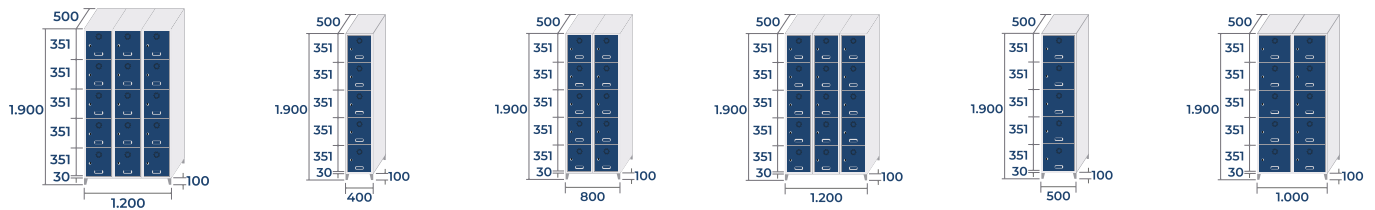
SP-30/4 73,2kg · 1,14m 3 SP-40/1 26kg · 0,38m 3 SP-40/2 46kg · 0,76m 3 SP-40/3 66kg · 1,14m 3 SP-50/1 28,8kg · 0,48m 3 SP-50/2 51,6kg · 0,95m 3
