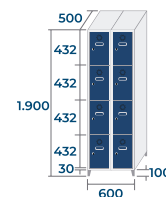
SC-30/2 37,1kg · 0,57m 3
