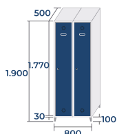
SV-40/2 45kg · 0,76m 3
