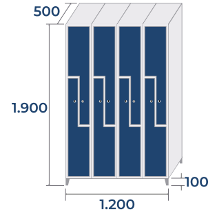
SL-30/4 69,1kg · 1,08m 3
