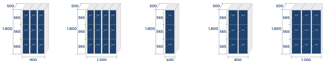
ECOM-30/3 PRO 51,6kg . 0,81m 3 ECOM-30/4 PRO 66,8kg . 1,08m 3 ECOM-40/1 PRO 24,2kg . 0,36m 3 ECOM-40/2 PRO 42,4kg . 0,72m 3 ECOM-40/3 PRO 60,6kg . 1,08m 3
