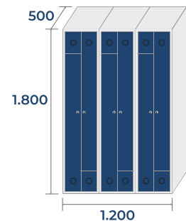
ECOL-40/3 PRO 72,3kg · 1,08m 3
