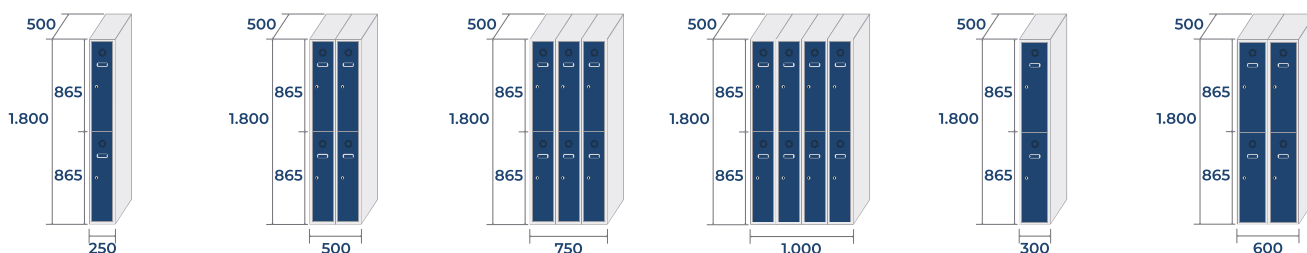
ECOT-25/1 PRO 18,4kg · 0,22m 3 ECOT-25/2 PRO 31,3kg · 0,45m 3 ECOT-25/3 PRO 44,2kg · 0,67m 3 ECOT-25/4 PRO 57,1kg · 0,9m 3 ECOT-30/1 PRO 19,1kg · 0,27m 3 ECOT-30/2 PRO 33,2kg · 0,54m 3
