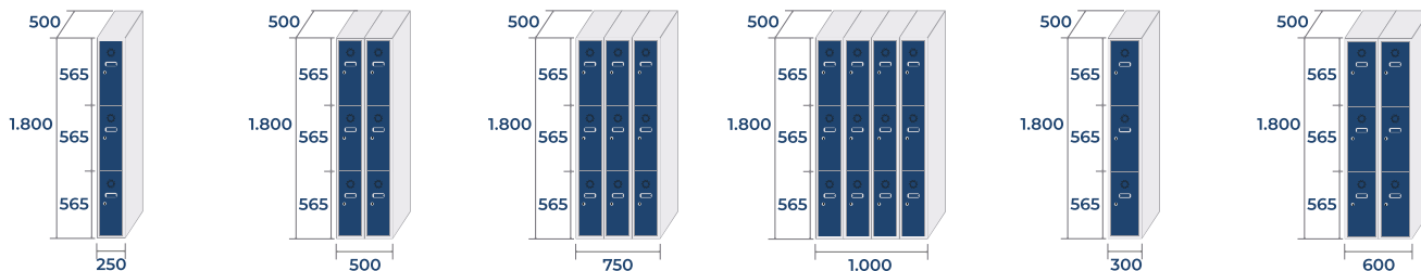
ECOM-25/1 PRO 19,9kg . 0,22m 3 ECOM-25/2 PRO 33,8kg . 0,45m 3 ECOM-25/3 PRO 47,7kg . 0,67m 3 ECOM-25/4 PRO 61,6kg . 0,9m 3 ECOM-30/1 PRO 21,2kg . 0,27m 3 ECOM-30/2 PRO 36,4kg . 0,54m 3
