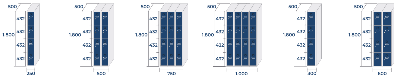
ECOC-25/1 PRO 20,8kg . 0,22m 3 ECOC-25/2 PRO 35,6kg . 0,45m 3 ECOC-25/3 PRO 50,4kg . 0,67m 3 ECOC-25/4 PRO 65,2kg . 0,9m 3 ECOC-30/1 PRO 22,3kg . 0,27m 3 ECOC-30/2 PRO 38,6kg . 0,54m 3
