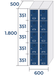
ECOP-30/2 PRO 40,9kg · 0,54m 3
