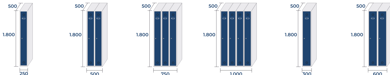
ECOV-25/1 PRO 16,7kg · 0,22m 3 ECOV-25/2 PRO 27,9kg · 0,45m 3 ECOV-25/3 PRO 39,1kg · 0,67m 3 ECOV-25/4 PRO 50,3kg · 0,9m 3 ECOV-30/1 PRO 19kg · 0,27m 3 ECOV-30/2 PRO 30,2kg · 0,54m 3
