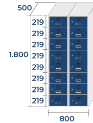
ECOZ-40/2 PRO 56,8kg · 0,72m 3
