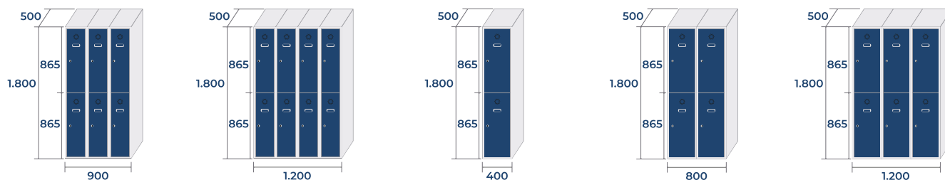
ECOT-30/3 PRO 47,3kg · 0,81m 3 ECOT-30/4 PRO 61,4kg · 1,08m 3 ECOT-40/1 PRO 23kg · 0,36m 3 ECOT-40/2 PRO 41kg · 0,72m 3 ECOT-40/3 PRO 59kg · 1,08m 3
