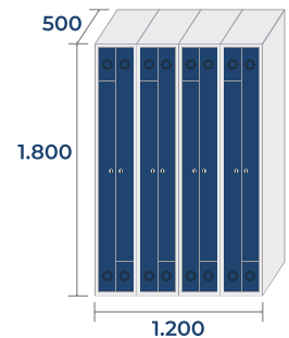
ECOL-30/4 PRO 79,8kg · 1,08m 3
