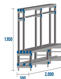
BANC-3-PVC-2000 28kg · 0,61m 3 · 8 ↓
