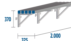
BANC-PARED-PVC-2000 15kg · 0,24m 3
