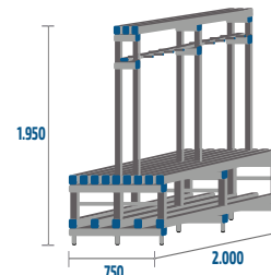
BANC-3-PVC-2000-DC 52kg · 1,02m 3 · 16 ↓
