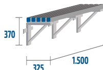
BANC-PARED-PVC-1500 12kg · 0,18m 3
