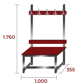
BANC-2-1000-FEN-INOX 24kg · 0,23m 3 · 5 ↓
