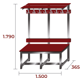
BANC-3-1500-FEN-INOX 38,5kg · 0,3m 3 · 8 ↓
