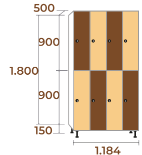
MHT-30/4 | MHFT-30/4 101kg | 110kg . 1,07m 3
