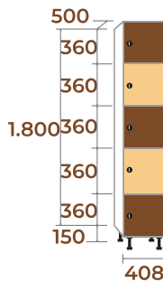
MHP-40/1 | MHFP-40/1 44kg | 47kg . 0,28m 3
