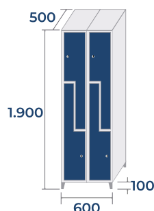
SL2-30/2 37,1kg · 0,54m 3
