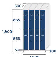
ST-25/4 56,6kg · 0,95m 3
